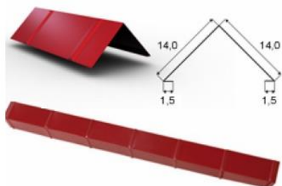
Zakończenie gąsiora dachowego
